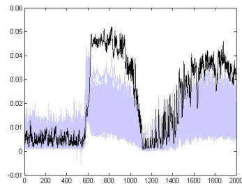
(d) MIA (param.) attack with 1024 traces.
